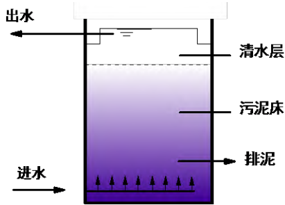
图 2 升流式水解酸化反应器结构示意图
